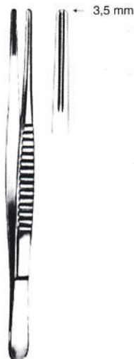
DE BAKEY 12310-16 16 cm 12310-20 20 cm 12310-24 24 cm 12310-30 30 cm
